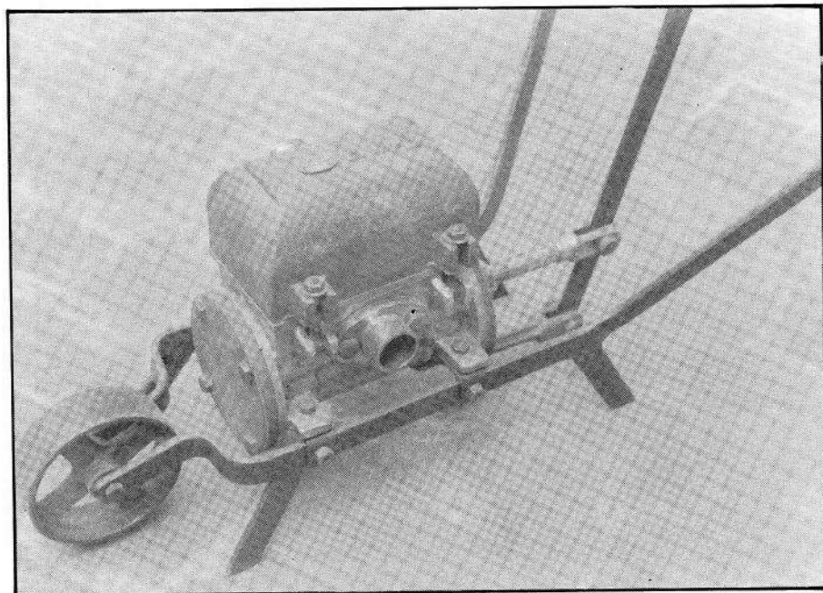
Les bombes de trasbalsar es començaren a fer servir els anys 1915-1920 i han arribat a l'actualitat. En un primer moment s'havien d'anar a buscar a Vilafranca o Molins de Rei. (fotografia feta del fons del Museu.)
